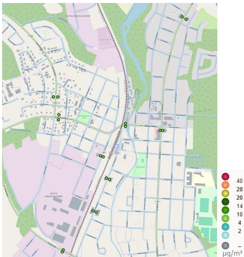
Figur 8. Beräknade halter av partiklar (PM 10 ) som årsmedelvärden i Aneby 2023.
