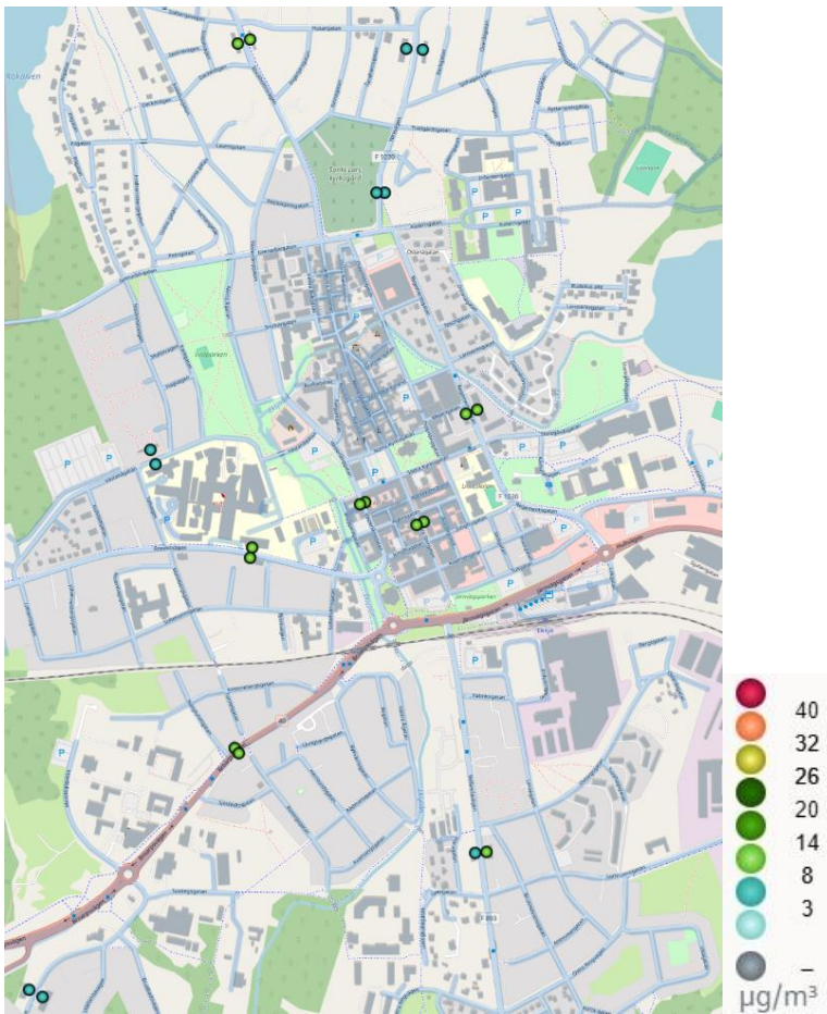
Figur 16. Beräknade halter av kvävedioxid (NO 2 ) som årsmedelvärden i Eksjö 2023.
