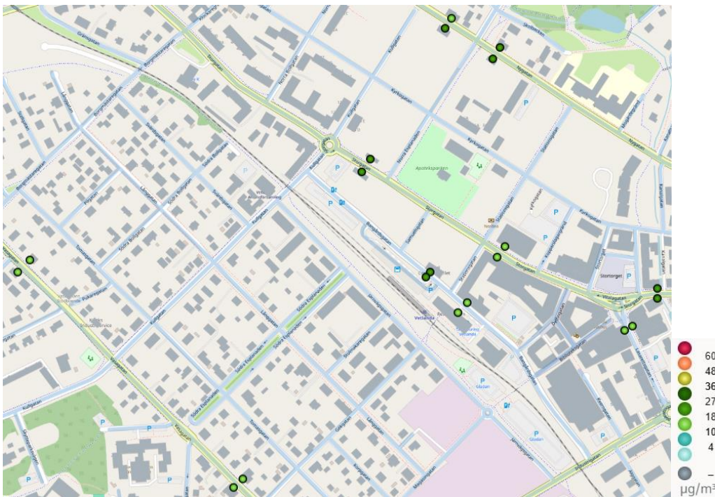
Figur 77. Beräknade halter av kvävedioxid (NO 2 ) som dygnsmedelvärden (98-percentil) i Vetlanda 2023.
