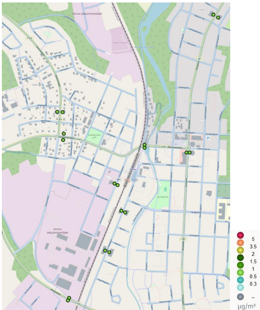
Figur 13. Beräknade halter av Bensen som årsmedelvärden i Aneby 2023.
