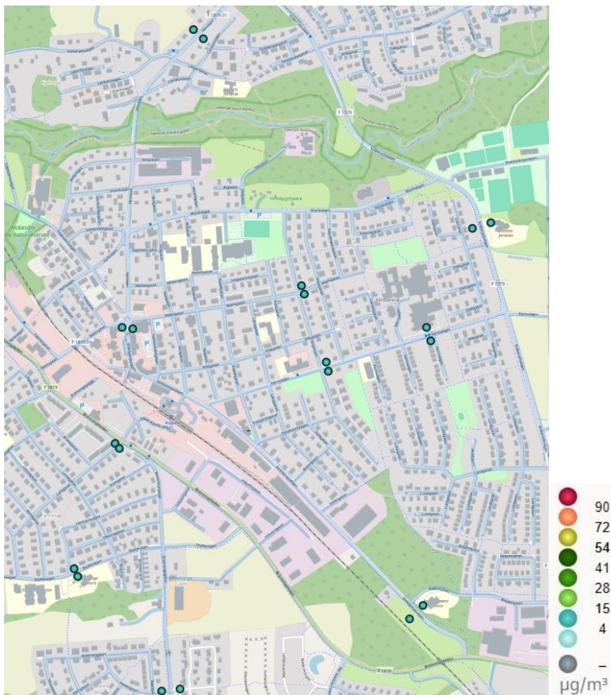
Figur 36. Beräknade halter av kvävedioxid (NO 2 ) som timmedelvärden (98-percentil) i Habo 2023.
