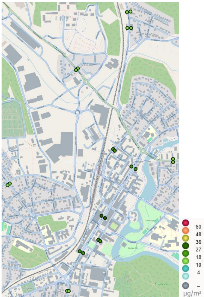
Figur 65. Beräknade halter av kvävedioxid (NO 2 ) som dygnsmedelvärden (98-percentil) i Tranås 2023.
