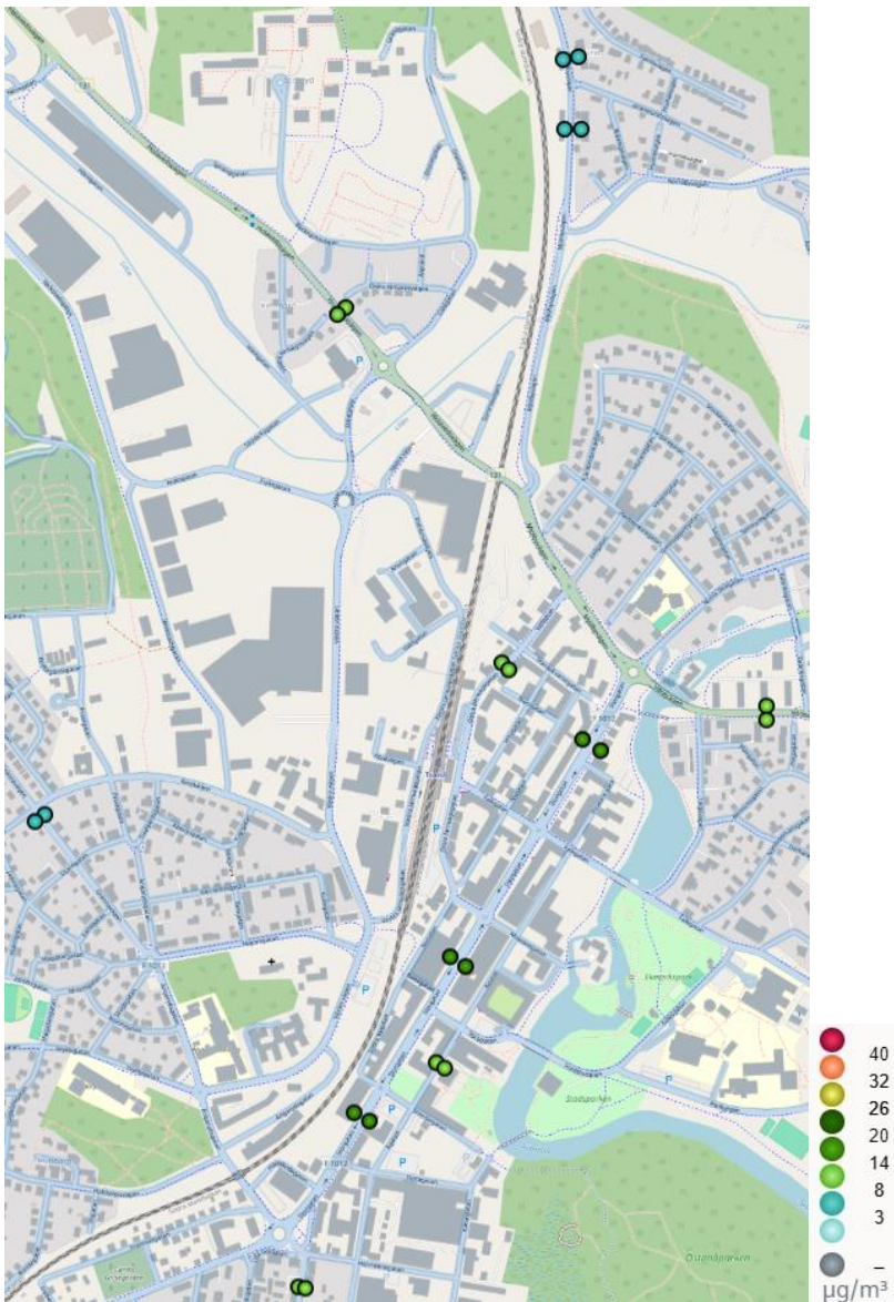
Figur 64. Beräknade halter av kvävedioxid (NO 2 ) som årsmedelvärden i Tranås 2023.
