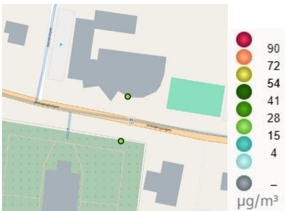
Figur 60. Beräknade halter av kvävedioxid (NO 2 ) som timmedelvärden (98-percentil) i Sävsjö 2023. Övre bild: Sävsjö. Nedre bild: Vrigstad
