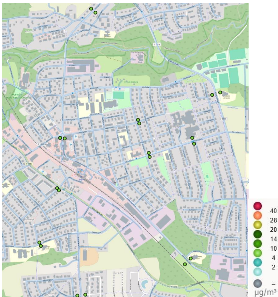
Figur 32. Beräknade halter av partiklar (PM 10 ) som årsmedelvärden i Habo 2023.
