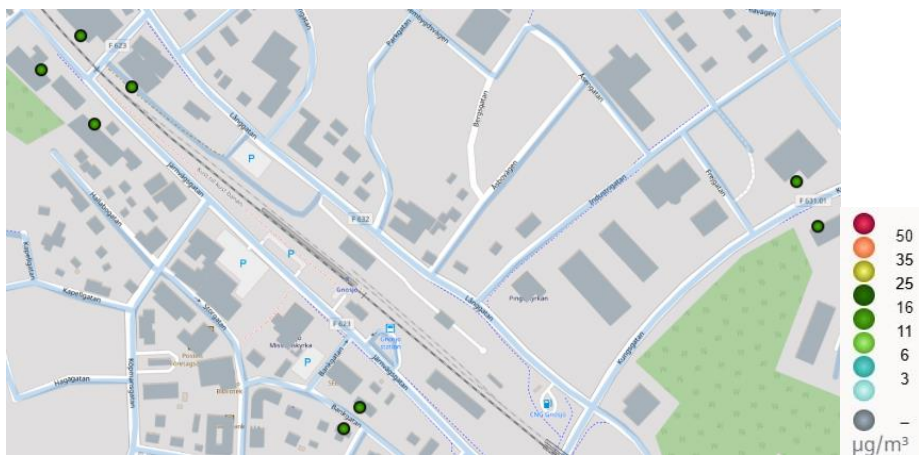
Figur 27. Beräknade halter av partiklar (PM 10 ) som dygnsmedelvärden (90-percentil) i Gnosjö 2023.
