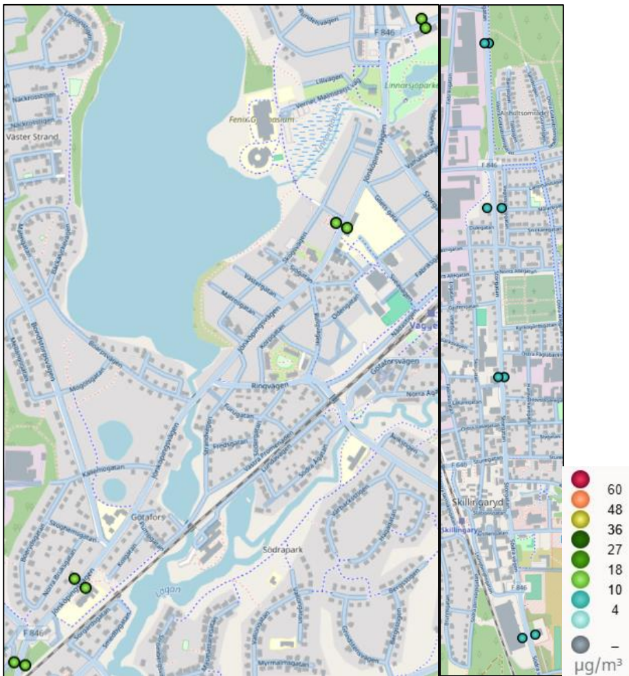
Figur 71. Beräknade halter av kvävedioxid (NO 2 ) som dygnsmedelvärden (98-percentil) i Vaggeryd-Skillingaryd 2023.
