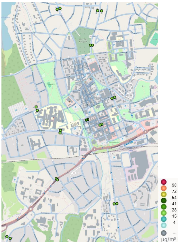
Figur 18. Beräknade halter av kvävedioxid (NO 2 ) som timmedelvärden (98-percentil) i Eksjö 2023.
