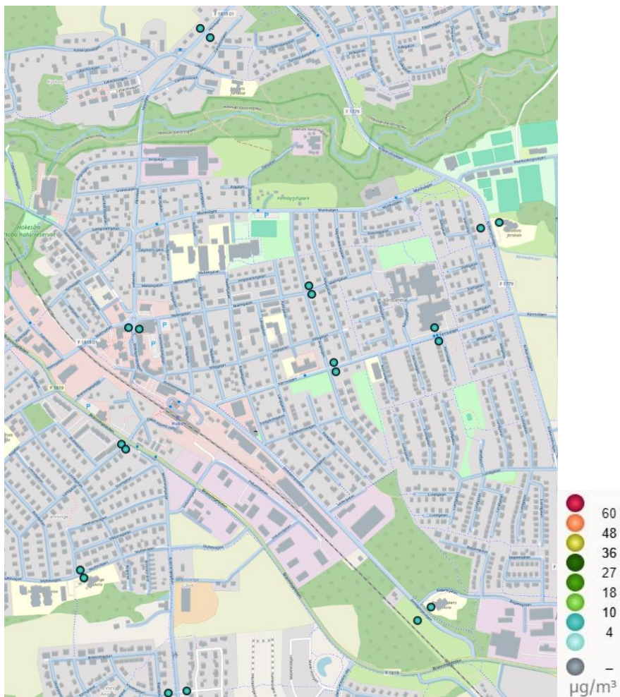
Figur 35. Beräknade halter av kvävedioxid (NO 2 ) som dygnsmedelvärden (98-percentil) i Habo 2023.
