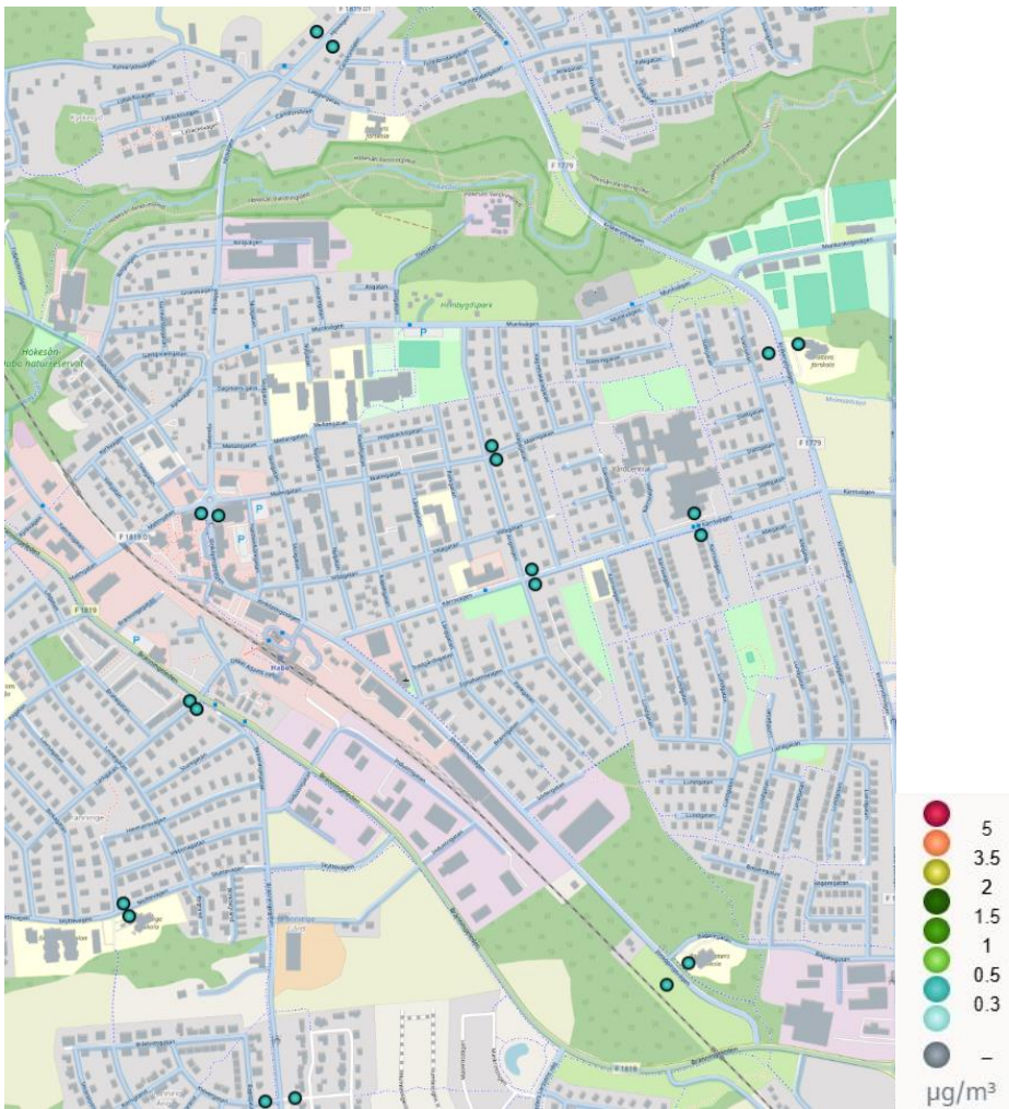
Figur 37. Beräknade halter av bensen som årsmedelvärden i Habo 2023.
