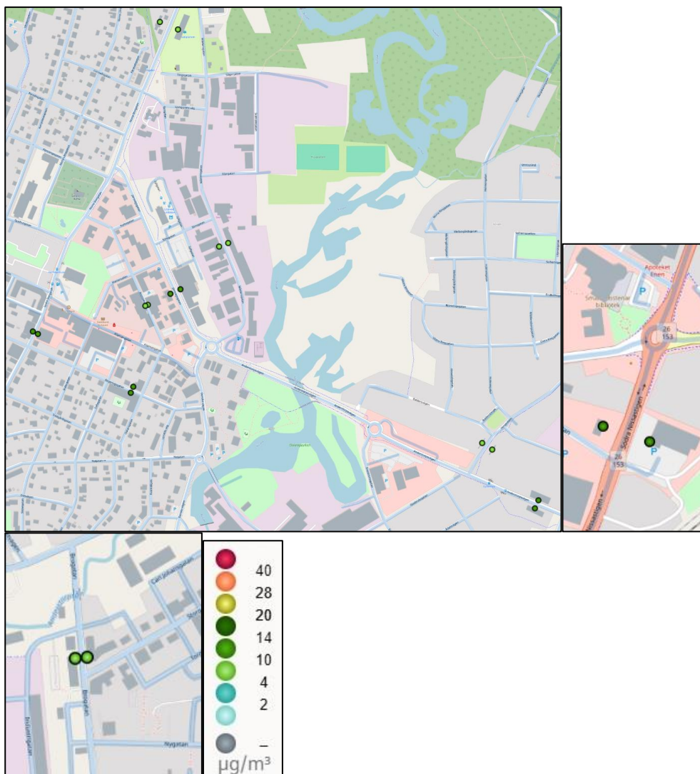
Figur 20. Beräknade halter av partiklar (PM 10 ) som årsmedelvärden i Gislaved 2023. Övre vänster: Gislaved. Nedre vänster: Smålandsstenar. Nedre högre: Anderstorp
