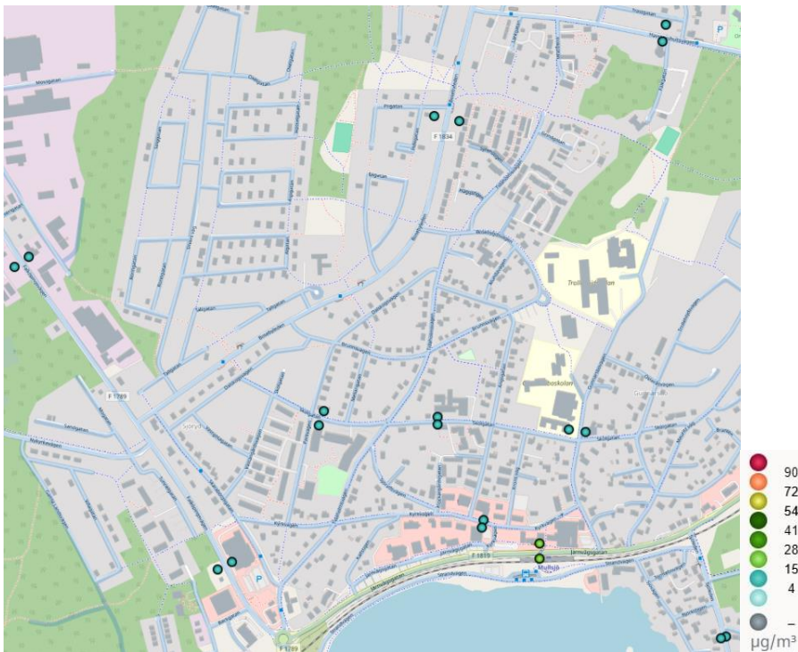
Figur 48. Beräknade halter av kvävedioxid (NO 2 ) som timmedelvärden (98-percentil) i Mullsjö 2023.
