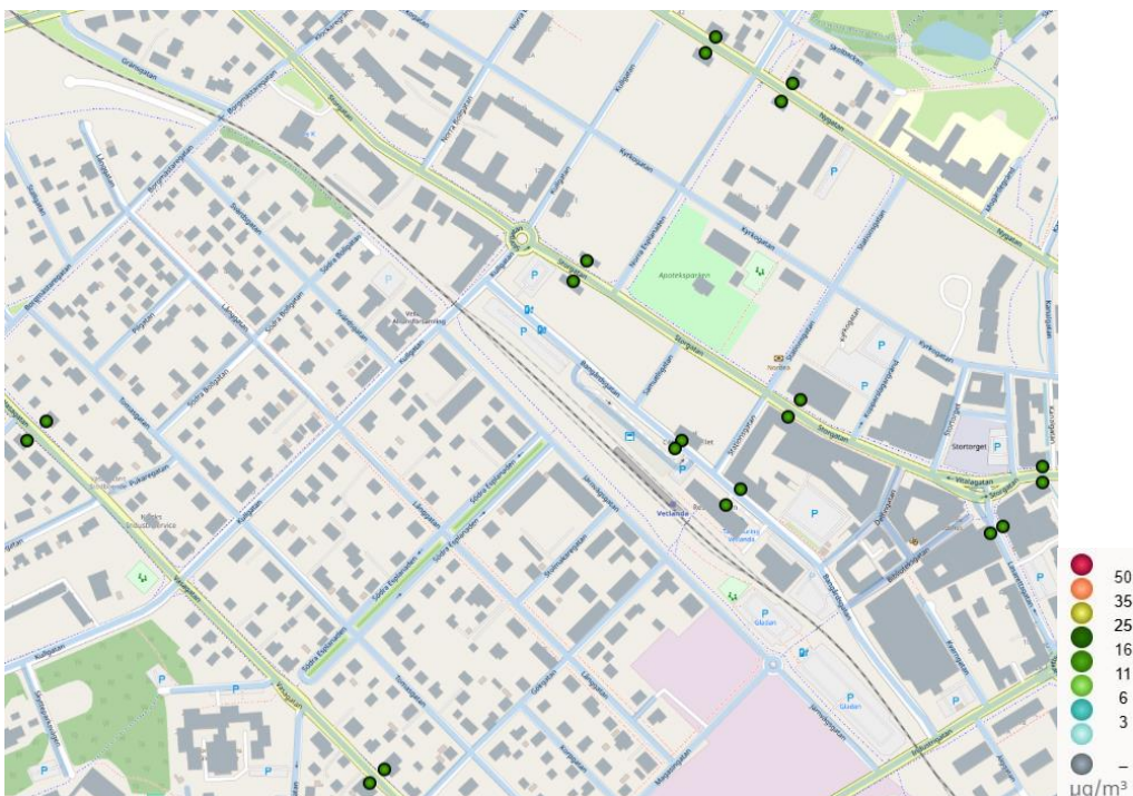
Figur 75. Beräknade halter av partiklar (PM 10 ) som dygnsmedelvärden (90-percentil) i Vetlanda 2023.
