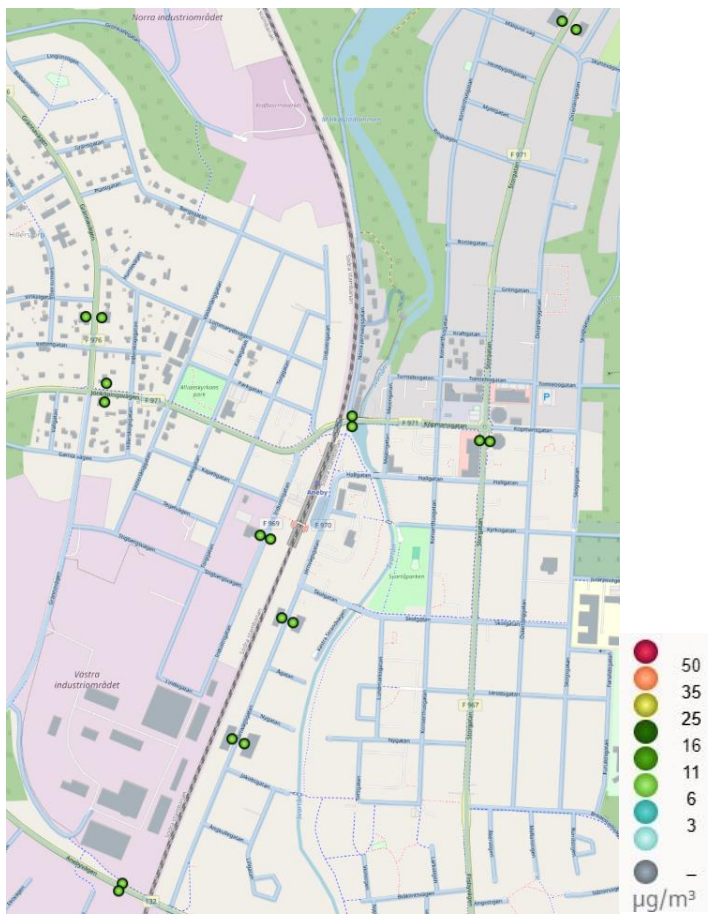
Figur 9. Beräknade halter av partiklar (PM 10 ) som dygnsmedelvärden (90-percentil) i Aneby 2023.
