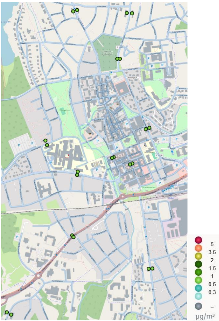
Figur 19. Beräknade halter av Bensen som årsmedelvärden i Eksjö 2023.
