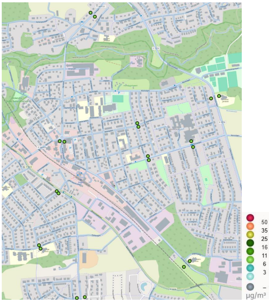
Figur 33. Beräknade halter av partiklar (PM 10 ) som dygnsmedelvärden (90-percentil) i Habo 2023.
