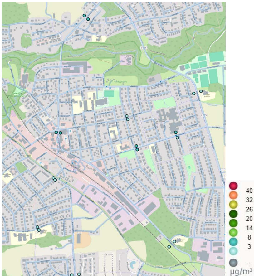
Figur 34. Beräknade halter av kvävedioxid (NO 2 ) som årsmedelvärden i Habo 2023.
