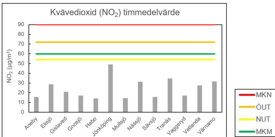
Figur 4. Högst beräknade halter av kvävedioxid som timmedelvärden (98-percentil) för respektive kommun
