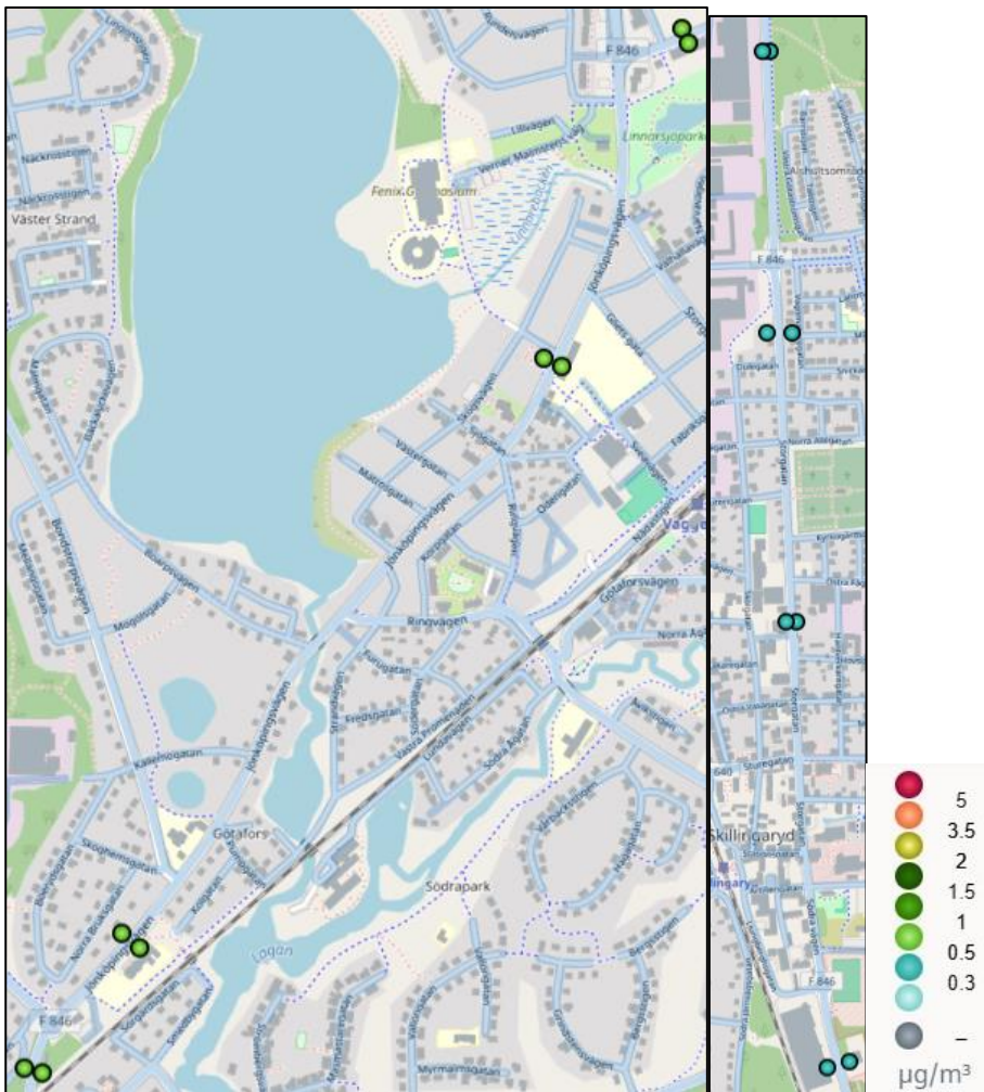
Figur 73. Beräknade halter av bensen som årsmedelvärden i Vaggeryd-Skillingaryd 2023.
