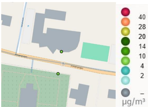
Figur 56. Beräknade halter av partiklar (PM 10 ) som årsmedelvärden i Sävsjö 2023. Övre bild: Sävsjö. Nedre bild: Vrigstad
