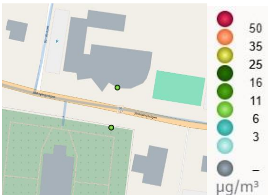
Figur 57. Beräknade halter av partiklar (PM 10 ) som dygnsmedelvärden (90-percentil) i Sävsjö 2023. Övre bild: Sävsjö. Nedre bild: Vrigstad
