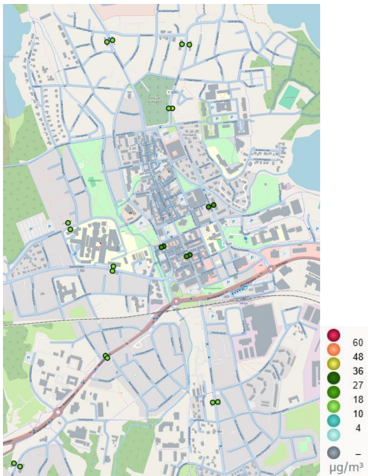
Figur 17. Beräknade halter av kvävedioxid (NO 2 ) som dygnsmedelvärden (98-percentil) i Eksjö 2023.
