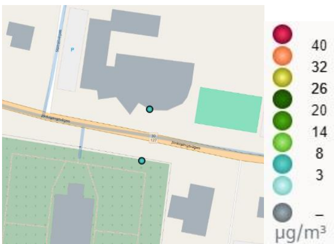
Figur 58. Beräknade halter av kvävedioxid (NO 2 ) som årsmedelvärden i Sävsjö 2023. Övre bild: Sävsjö. Nedre bild: Vrigstad
