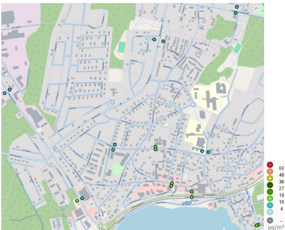
Figur 47. Beräknade halter av kvävedioxid (NO 2 ) som dygnsmedelvärden (98-percentil) i Mullsjö 2023.
