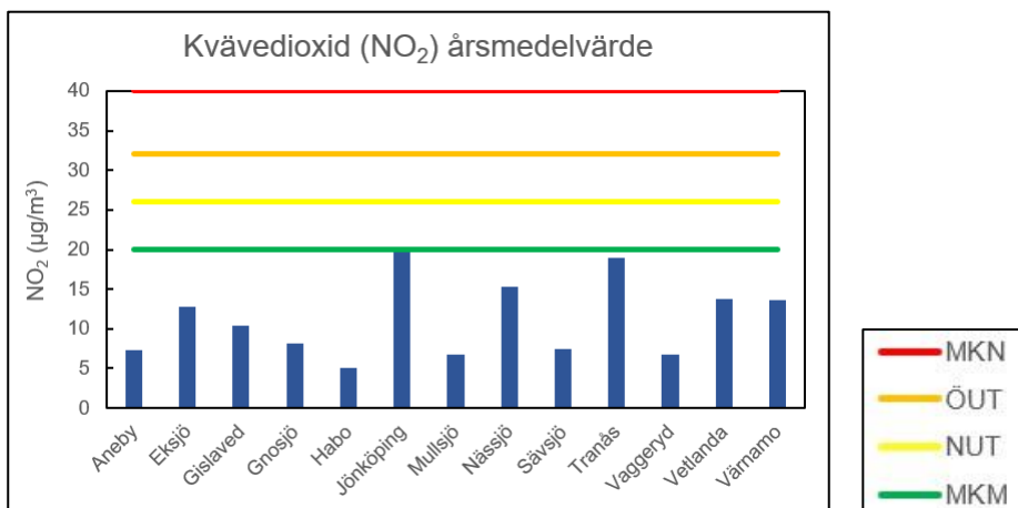
Figur 2. Högst beräknade halter av kvävedioxid som årsmedelvärden för respektive kommun
