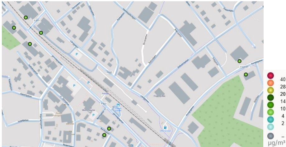
Figur 26. Beräknade halter av partiklar (PM 10 ) som årsmedelvärden i Gnosjö 2023.
