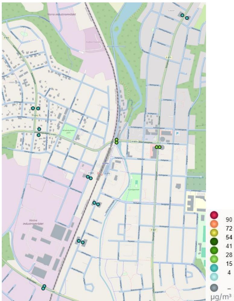
Figur 12. Beräknade halter av kvävedioxid (NO 2 ) som timmedelvärden (98-percentil) i Aneby 2023.
