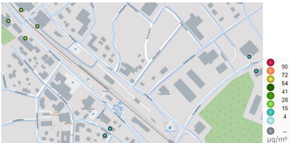
Figur 30. Beräknade halter av kvävedioxid (NO 2 ) som timmedelvärden (98-percentil) i Gnosjö 2023.
