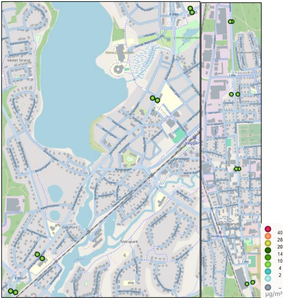
Figur 68. Beräknade halter av partiklar (PM 10 ) som årsmedelvärden i Vaggeryd-Skillingaryd 2023.
