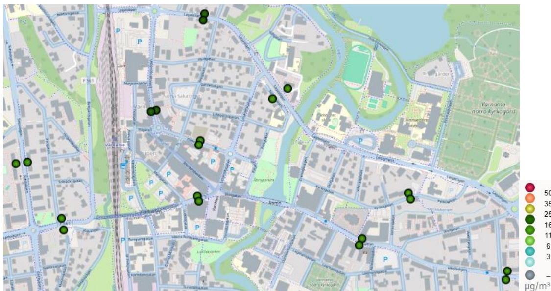
Figur 81. Beräknade halter av partiklar (PM 10 ) som dygnsmedelvärden (90-percentil) i Värnamo 2023.
