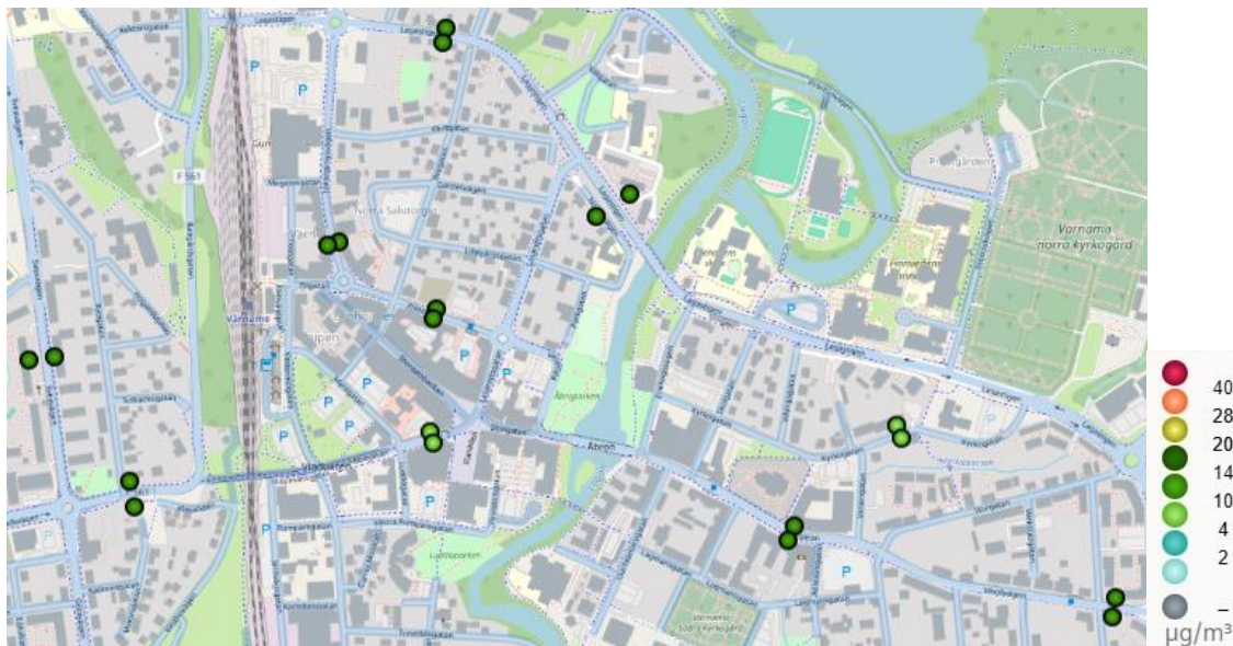
Figur 80. Beräknade halter av partiklar (PM 10 ) som årsmedelvärden i Värnamo 2023.
