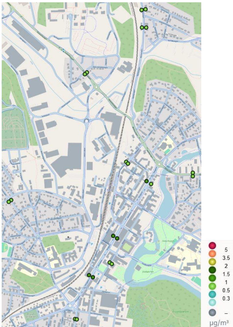
Figur 67. Beräknade halter av Bensen som årsmedelvärden i Tranås 2023.
