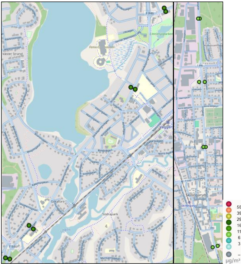
Figur 69. Beräknade halter av partiklar (PM 10 ) som dygnsmedelvärden (90-percentil) i Vaggeryd-Skillingaryd 2023.
