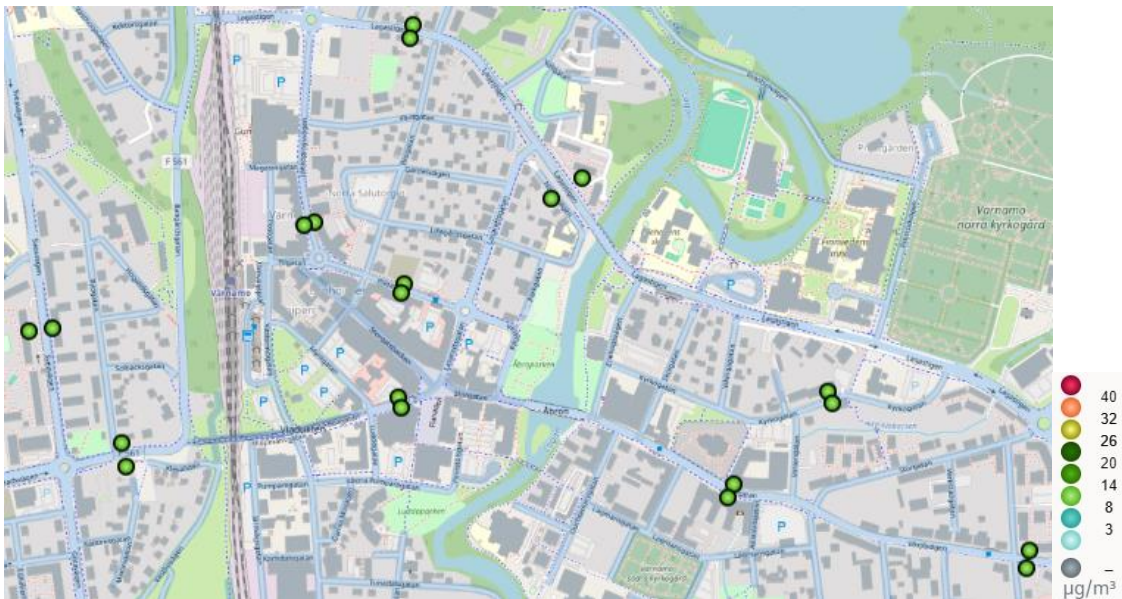
Figur 82. Beräknade halter av kvävedioxid (NO 2 ) som årsmedelvärden i Värnamo 2023.
