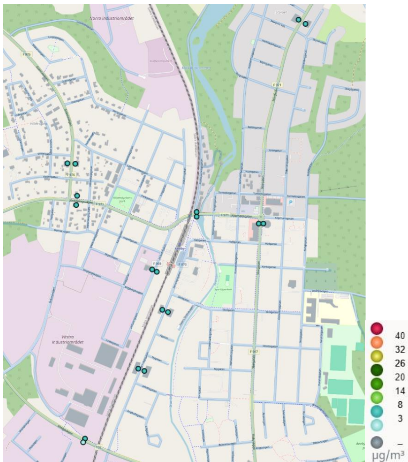
Figur 10. Beräknade halter av kvävedioxid (NO 2 ) som årsmedelvärden i Aneby 2023.
