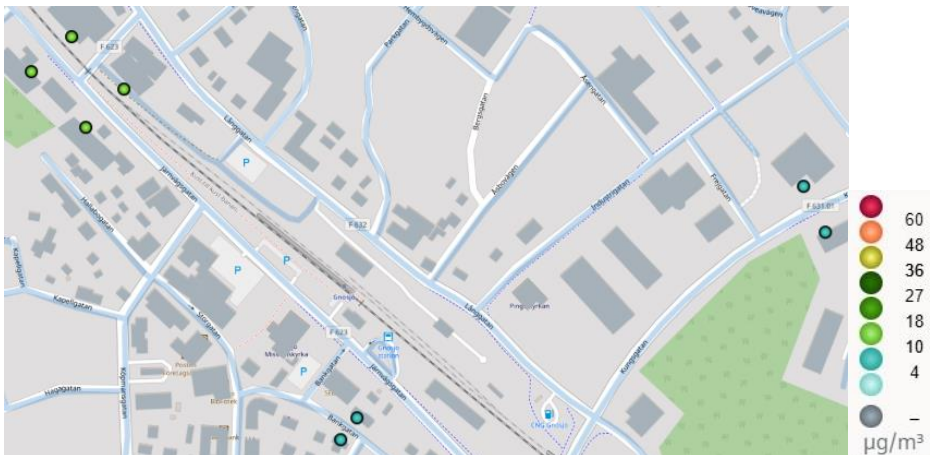
Figur 29. Beräknade halter av kvävedioxid (NO 2 ) som dygnsmedelvärden (98-percentil) i Gnosjö 2023.
