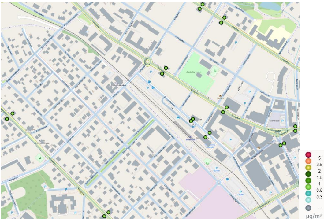
Figur 79. Beräknade halter av Bensen som årsmedelvärden i Vetlanda 2023.
