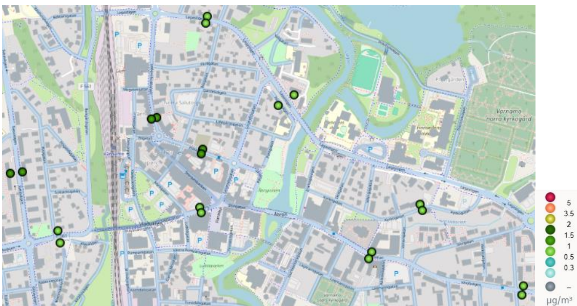
Figur 85. Beräknade halter av Bensen som årsmedelvärden i Värnamo 2023.
