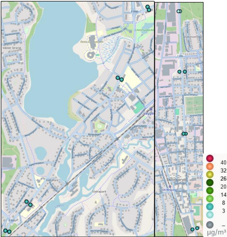
Figur 70. Beräknade halter av kvävedioxid (NO 2 ) som årsmedelvärden i Vaggeryd-Skillingaryd 2023.
