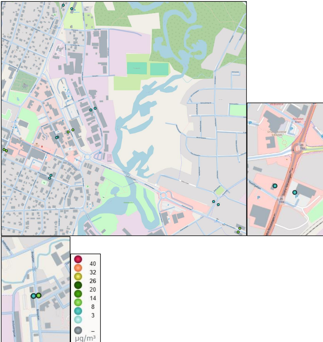
Figur 22. Beräknade halter av kvävedioxid (NO 2 ) som årsmedelvärden i Gislaved 2023. Övre vänster: Gislaved. Nedre vänster: Smålandsstenar. Nedre högre: Anderstorp
