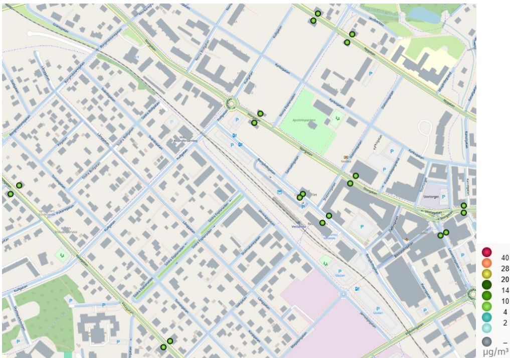
Figur 74. Beräknade halter av partiklar (PM 10 ) som årsmedelvärden i Vetlanda 2023.
