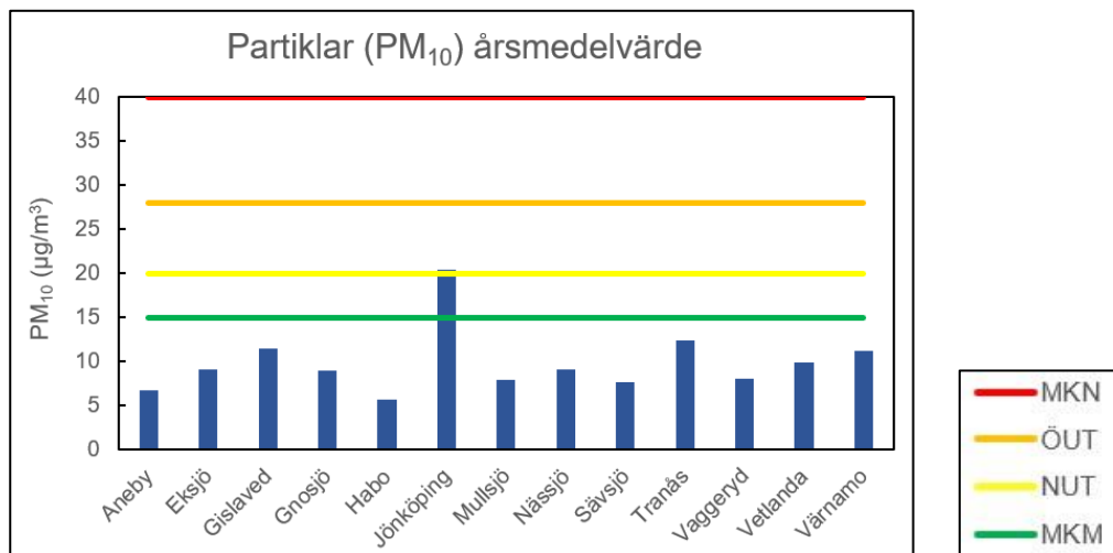
Figur 5. Högst beräknade halter av partiklar (PM 10 ) som årsmedelvärden för respektive kommun
