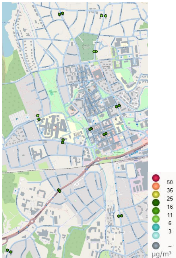
Figur 15. Beräknade halter av partiklar (PM 10 ) som dygnsmedelvärden (90-percentil) i Eksjö 2023.
