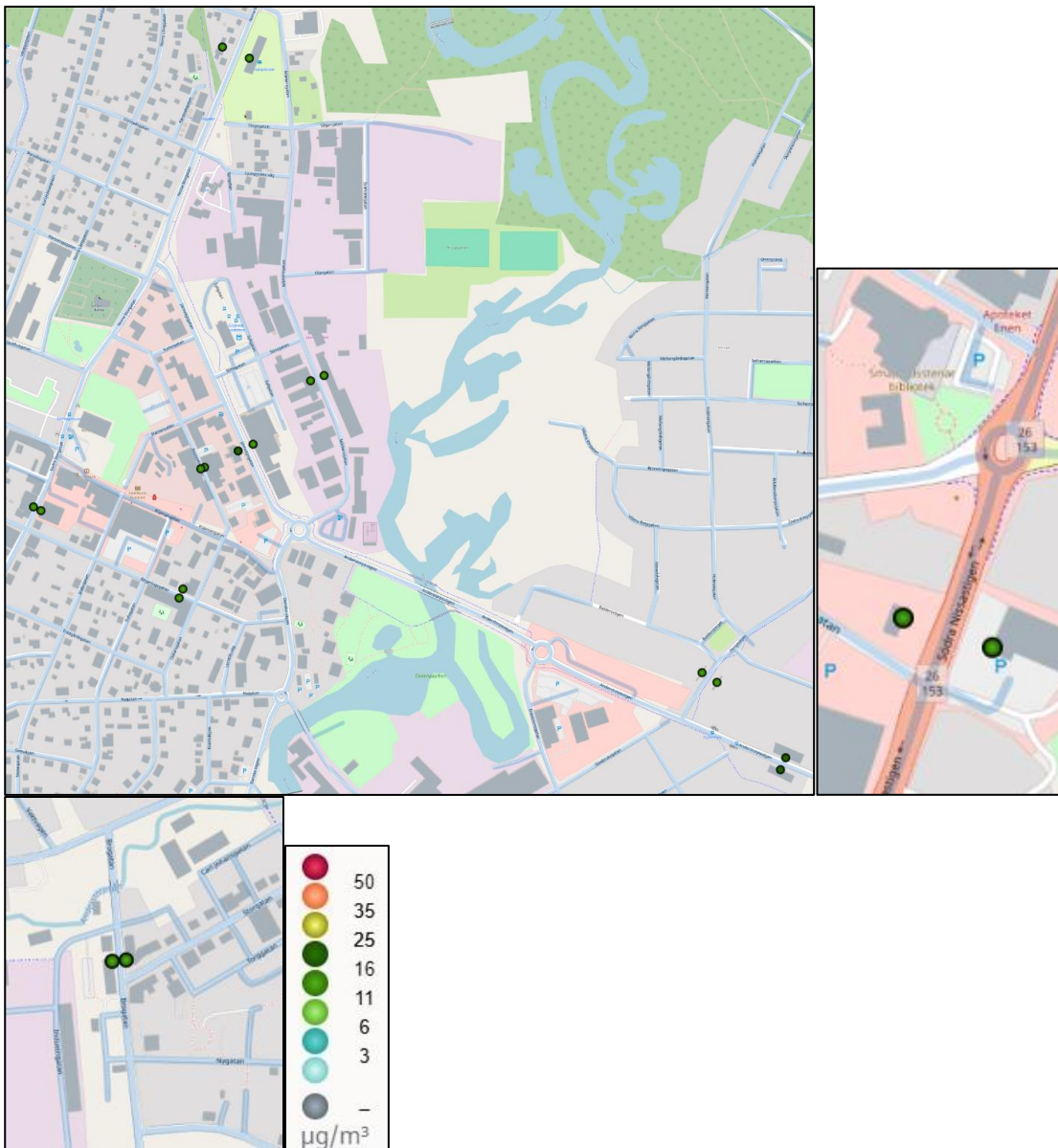
Figur 21. Beräknade halter av partiklar ( \text{PM}_{10} ) som dygnsmedelvärden (90-percentil) i Gislaved 2023. Övre vänster: Gislaved. Nedre vänster: Smålandsstenar. Nedre högre: Anderstorp
