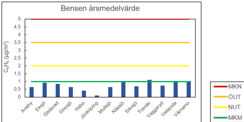
Figur 7. Högst beräknade halter av bensen som årsmedelvärden för respektive kommun
