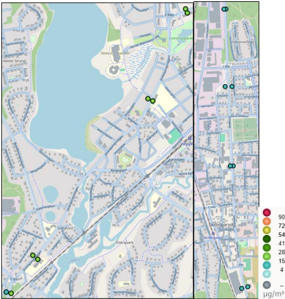
Figur 72. Beräknade halter av kvävedioxid (NO 2 ) som timmedelvärden (98-percentil) i Vaggeryd-Skillingaryd 2023.
