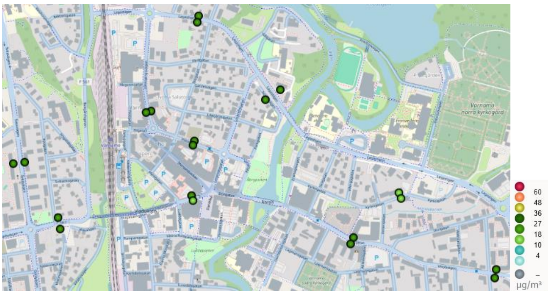
Figur 83. Beräknade halter av kvävedioxid (NO 2 ) som dygnsmedelvärden (98-percentil) i Värnamo 2023.
