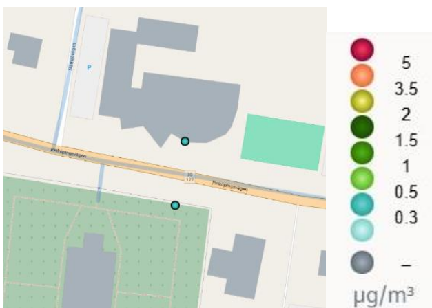
Figur 61. Beräknade halter av Bensen som årsmedelvärden i Sävsjö 2023. Övre bild: Sävsjö. Nedre bild: Vrigstad
