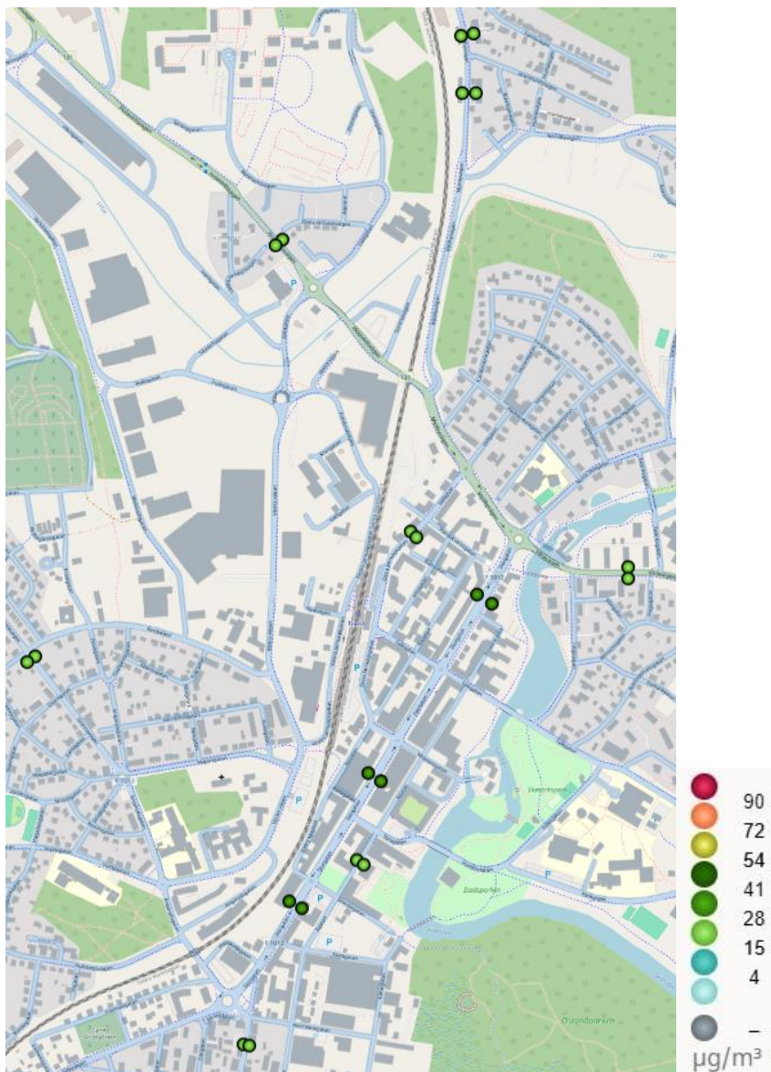
Figur 66. Beräknade halter av kvävedioxid (NO 2 ) som timmedelvärden (98-percentil) i Tranås 2023.
