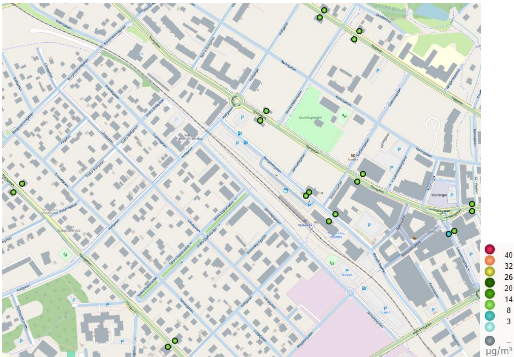
Figur 76. Beräknade halter av kvävedioxid (NO 2 ) som årsmedelvärden i Vetlanda 2023.
