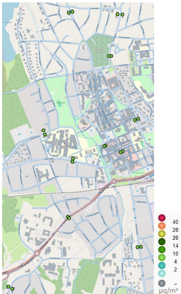
Figur 14. Beräknade halter av partiklar (PM 10 ) som årsmedelvärden i Eksjö 2023.
