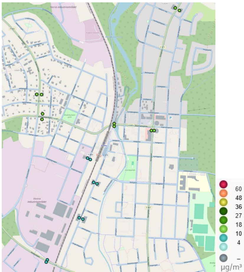
Figur 11. Beräknade halter av kvävedioxid (NO 2 ) som dygnsmedelvärden (98-percentil) i Aneby 2023.
