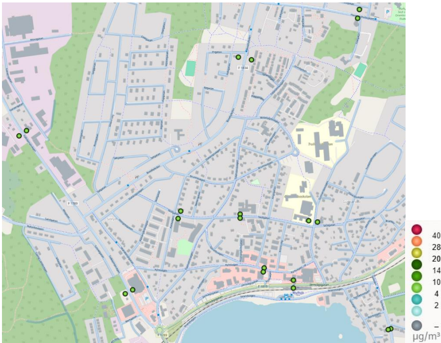
Figur 44. Beräknade halter av partiklar (PM 10 ) som årsmedelvärden i Mullsjö 2023.
