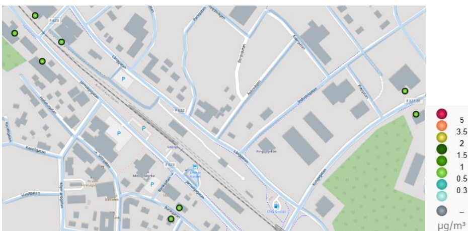
Figur 31. Beräknade halter av Bensen som årsmedelvärden i Gnosjö 2023.
